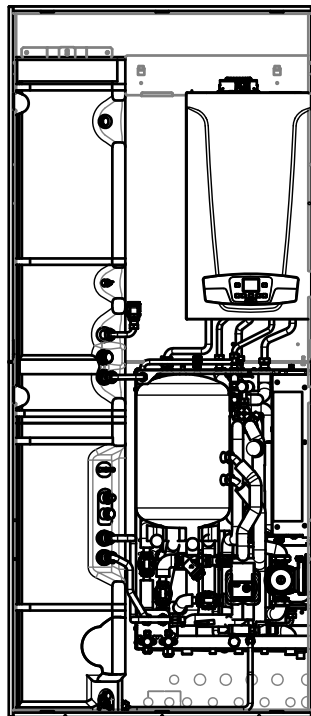
Sistema Ibrido integrato ad incasso con pompe di calore BAXI mod. CSI IN SPLIT H
