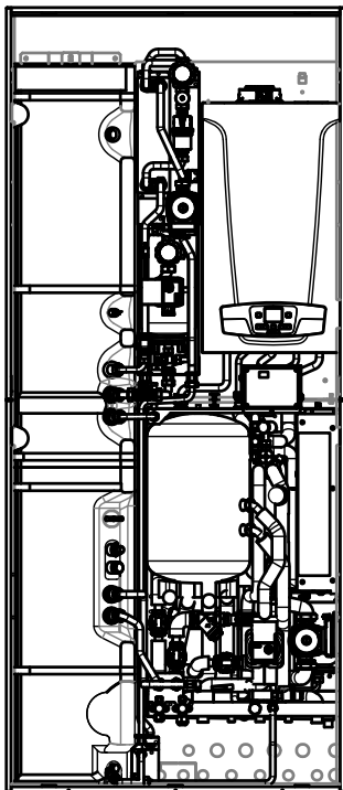
Sistema Ibrido integrato ad incasso con pompe di calore BAXI mod. CSI IN SPLIT H + Kit Solare
